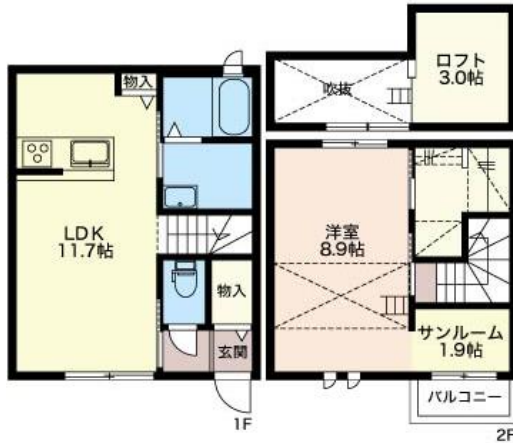
【間取図】
