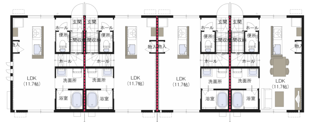
1階平面図
