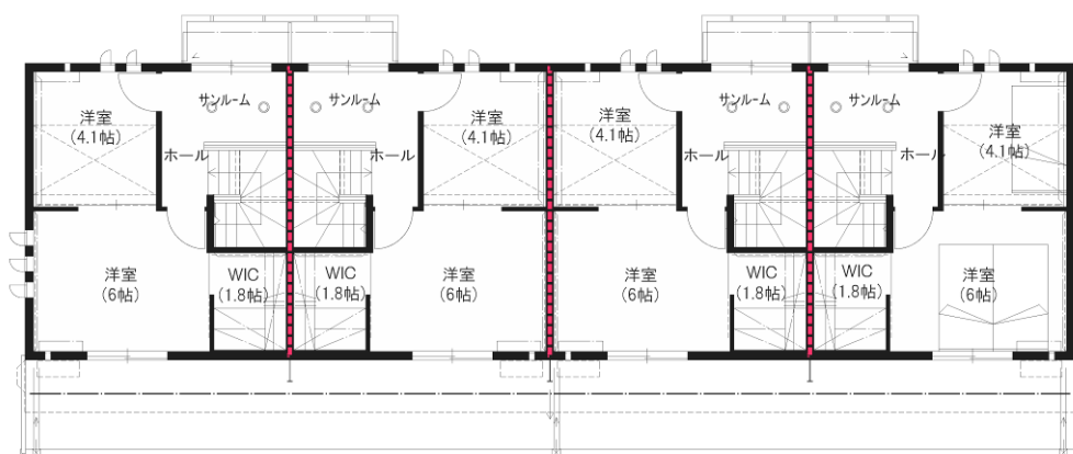
2階平面図
