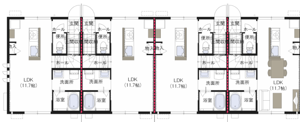
1階平面図
