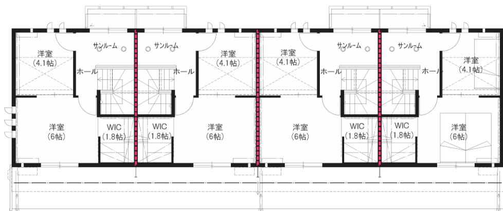
2階平面図
