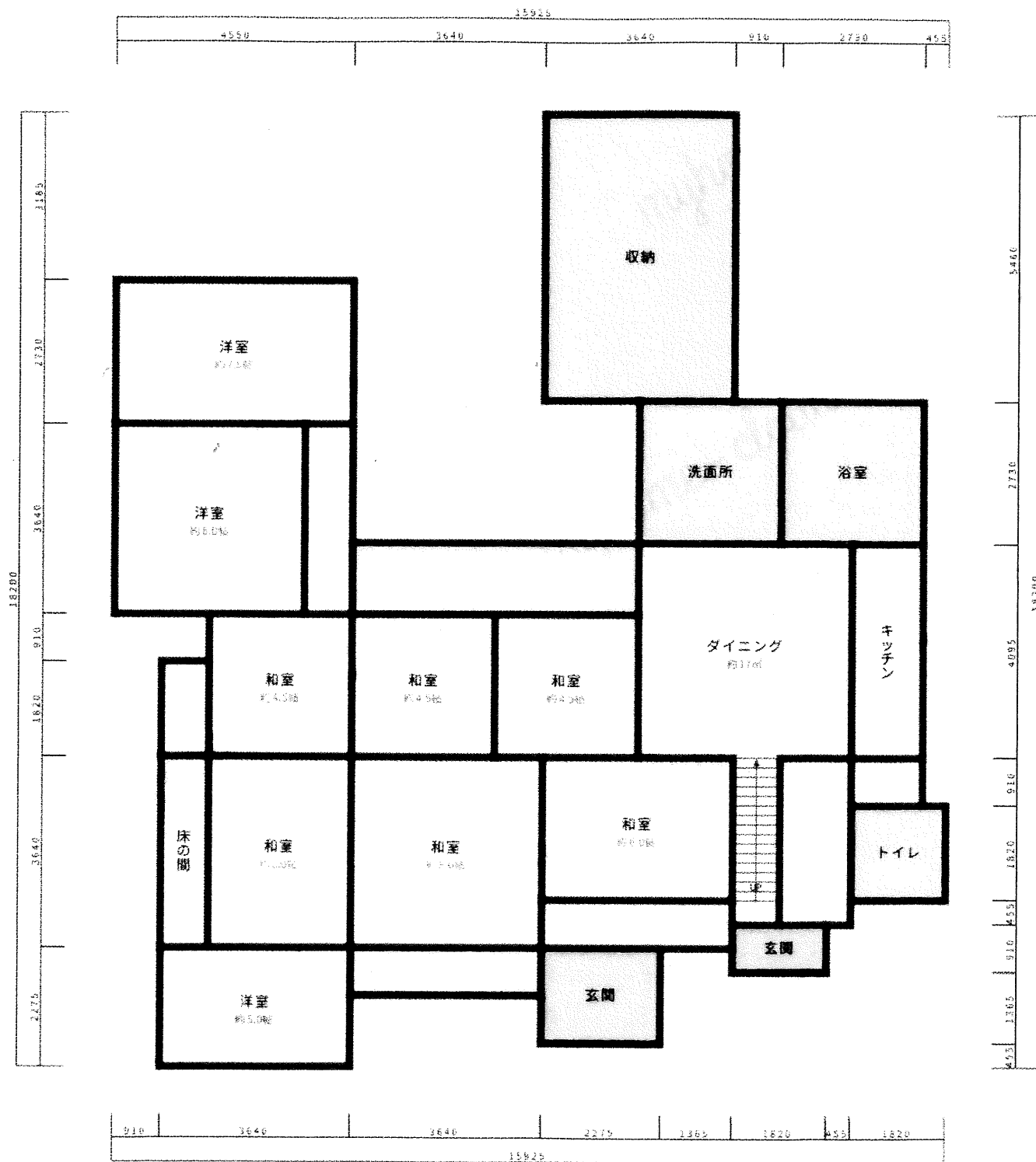
1階平面図
