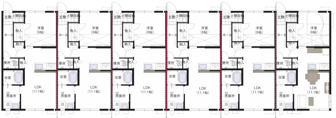
1階平面図
