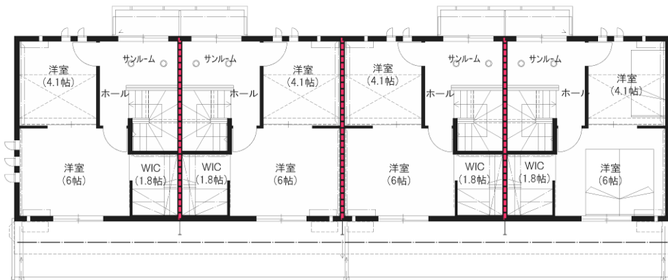
2階平面図
